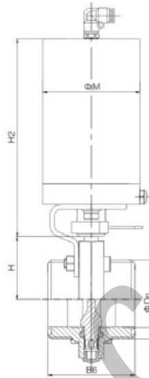
不锈钢气动蝶阀 SS Pneumatic butterfly valve NO.DS-VDF130Q1
