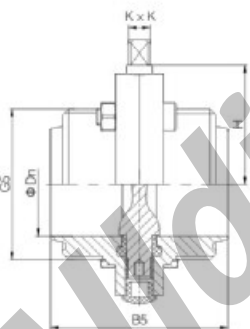
螺纹式MALE/MALE(RJT) NO.RJT-VDF130XX
